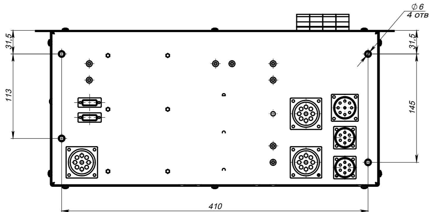
Вид снизу
